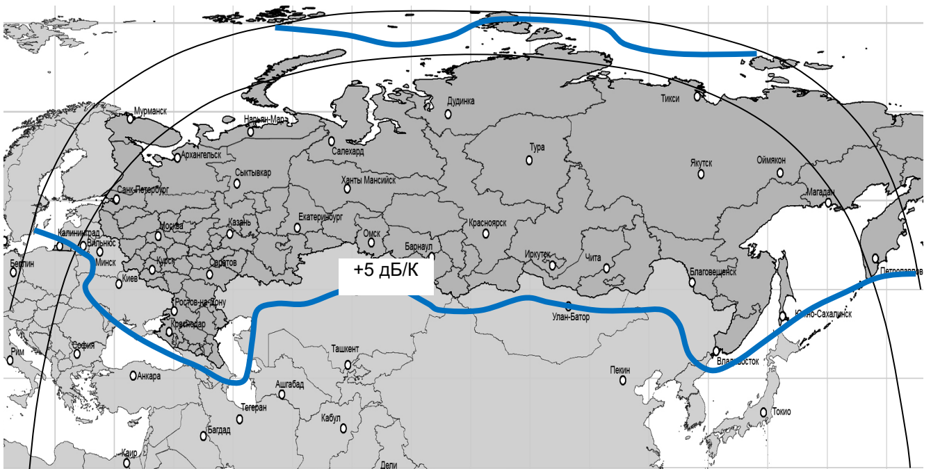
Рис. 2.5. Зона обслуживания Российского луча на прием (значения G/T)
