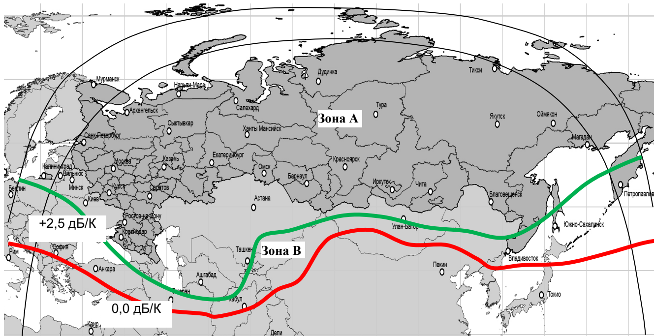
Рис. 2.1. Зона обслуживания в С-диапазоне на прием (значения G/T)
