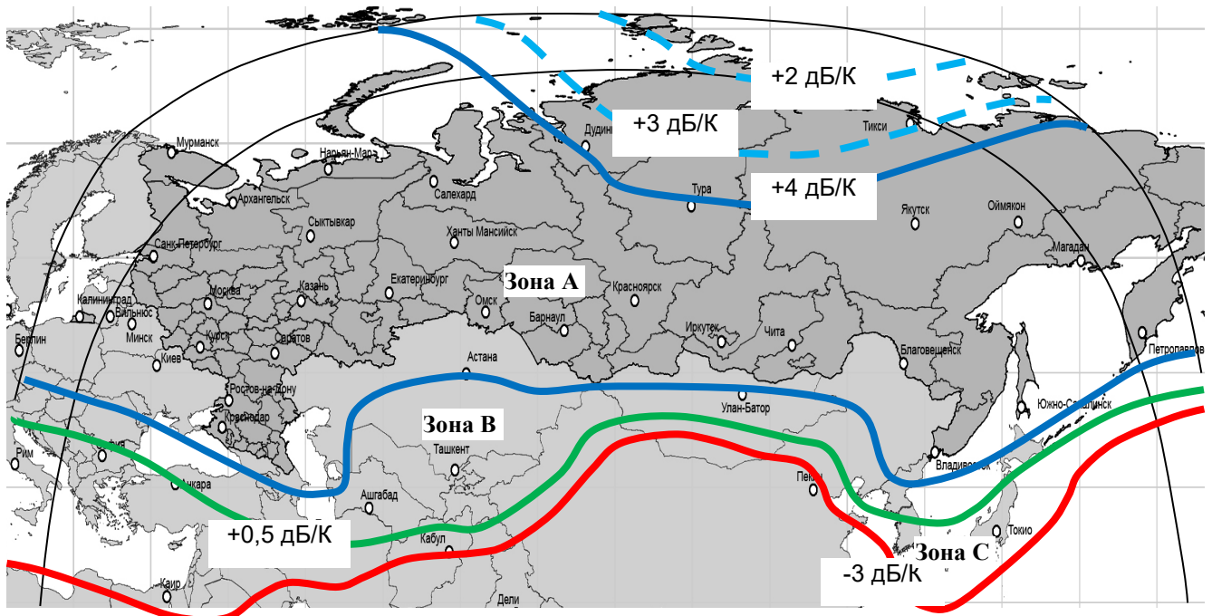
Рис. 2.4. Зона обслуживания Северного луча на прием (значения G/T)
