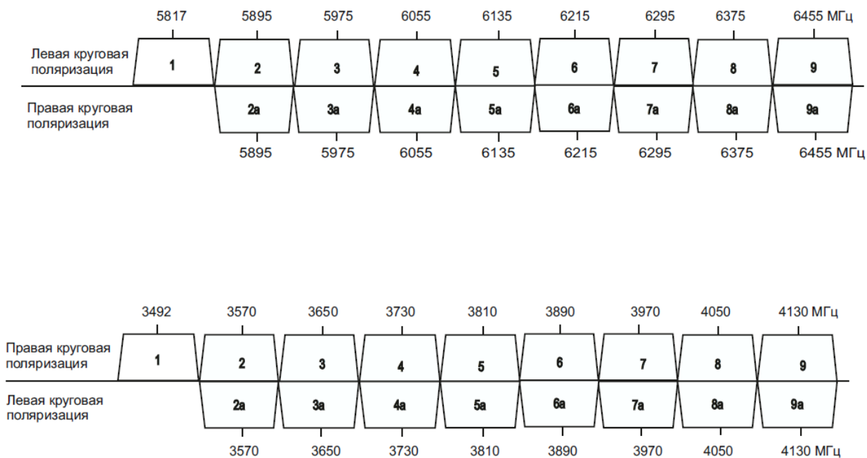
Рис. 2.3. Частотно-поляризационный план БРК С-диапазона
