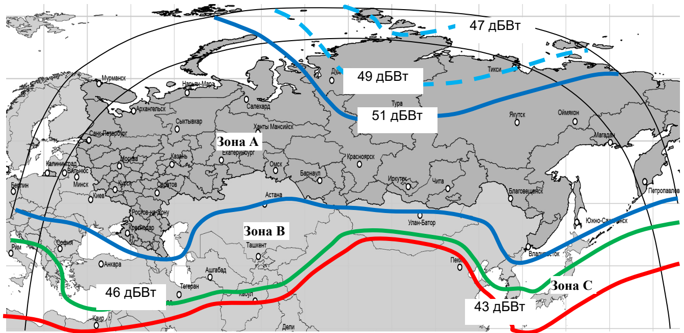
Рис. 2.6. Зона обслуживания Северного луча на передачу (значения ЭИИМ)
